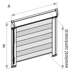
Rys. 2 Szerokość i wysokość całkowita rolety
